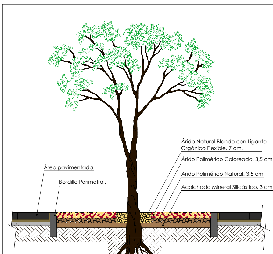
ALCORQUE DRENANTE de 10 cm. de ESPESOR, SISTEMA "Stone Drain®"
